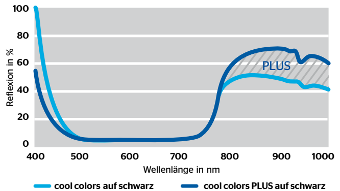
Theoretische Wirkungsweise cool colors und cool colors PLUS auf schwarzem Untergrund
