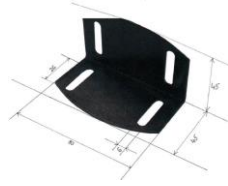
PRÍCHYTKA „L“ veľká
